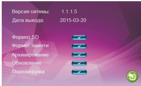
Рис.5 Меню "Информация"
